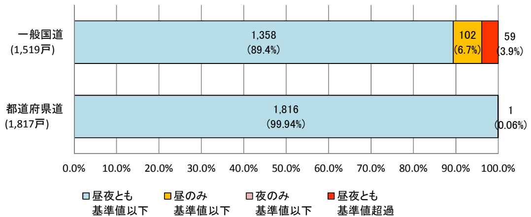
図 5.5 道路種類別の環境基準達成状況
