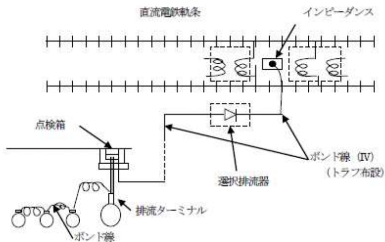
選択排流方式施工例
