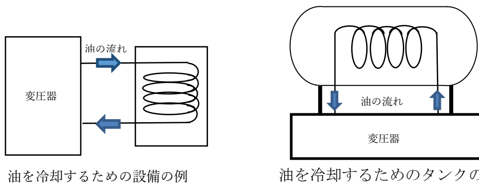
第4-14図 変圧器油を冷却するための付属設備
