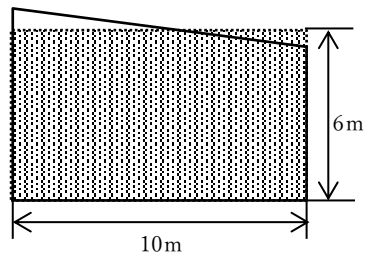
例3 給油空地が内在しない例
