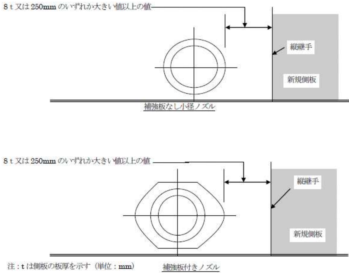
図4 側ノズルと側板継手の関係
