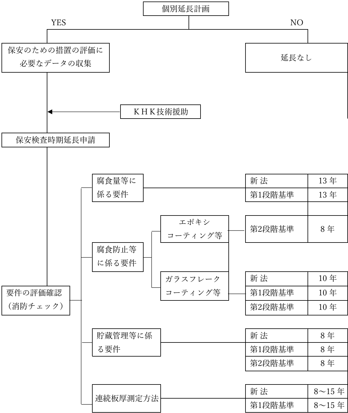
特定屋外タンク貯蔵所の保安検査の時期延長に係るフロー
