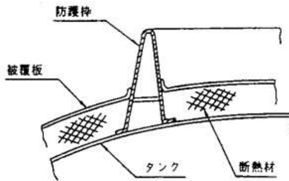
図 6-20 タンク胴板に直接取り付ける防護枠
