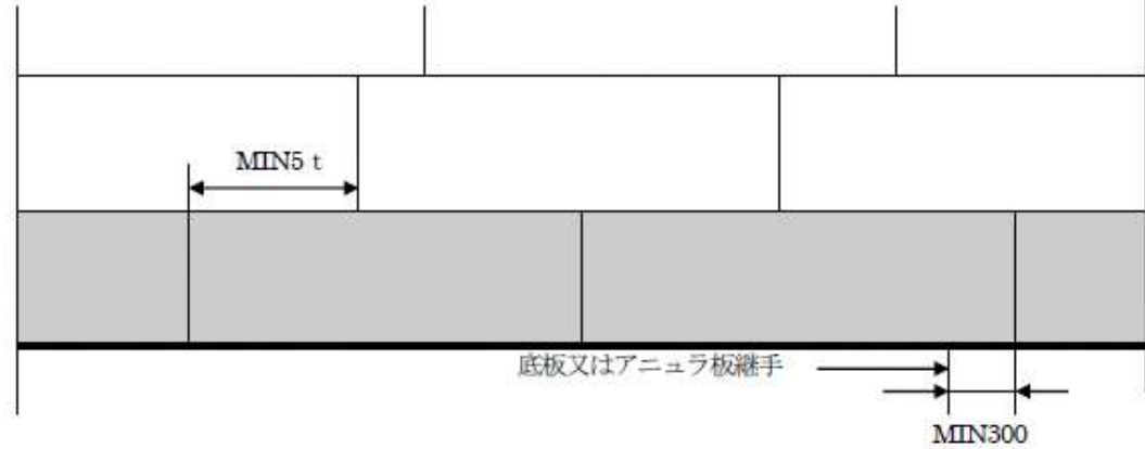
側板中段の取替
