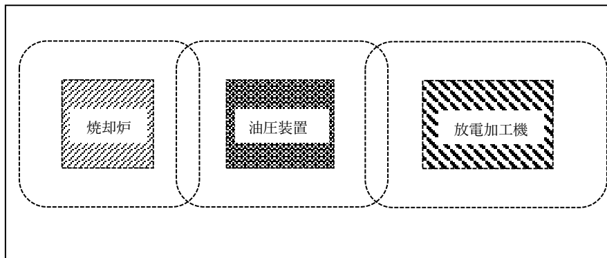
第4-6図 部分規制の一般取扱所と認めることができないものの例
