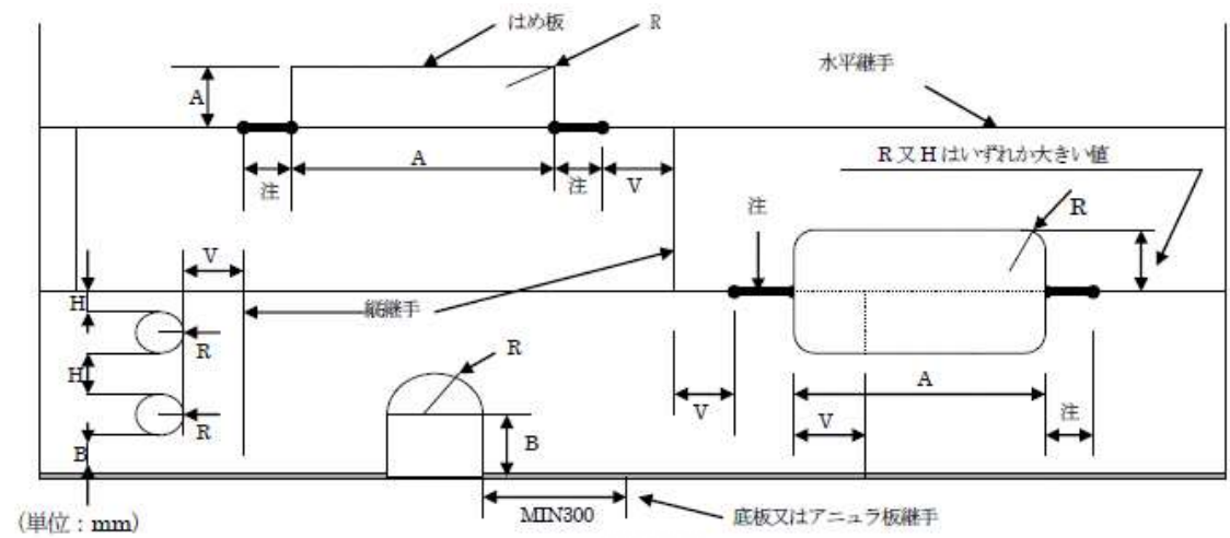
図5 側板のはめ板取付け
