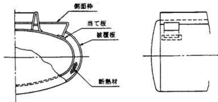
図 6-9 タンク胴板に直接取り付けする側面枠の方法
