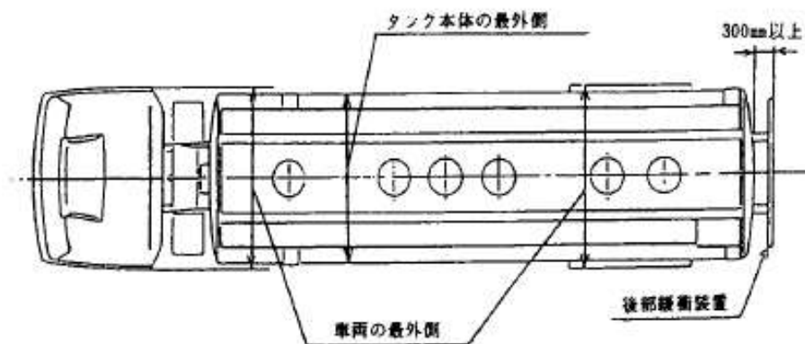
図6-29 最大容量が20klを超える移動タンク貯蔵所のタンクの位置
