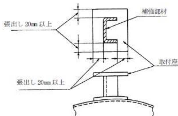
図 6-12 補強部材の取付座の大きさ
