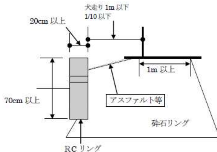
図-2 側板直下RCリング基礎
