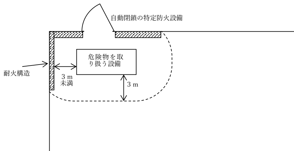
第4-17図 空地の保有例
