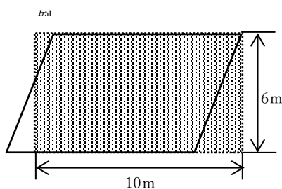
(例) 敷地と給油空地の関係
