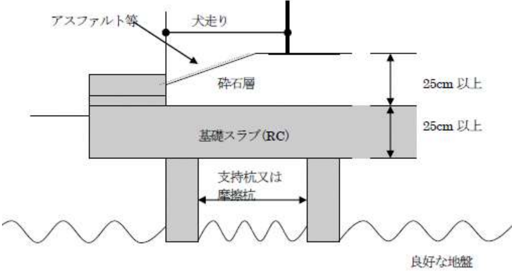
図－ 4 杭基礎
