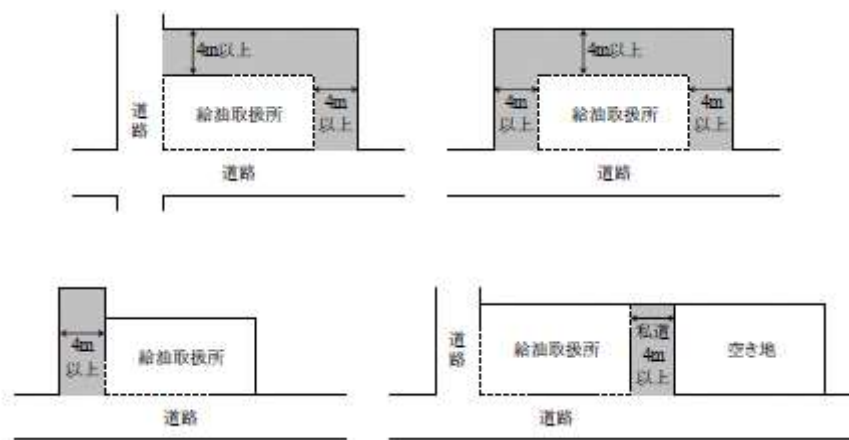
自動車が出入りする側の例
