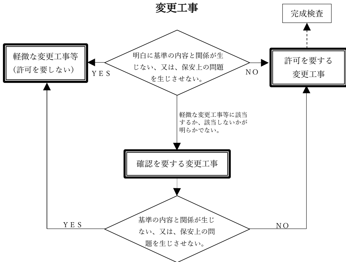
図1 製造所等において行われる変更工事に係る判断のフロー
