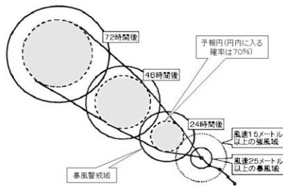
■ 台風の進路予想説明図
