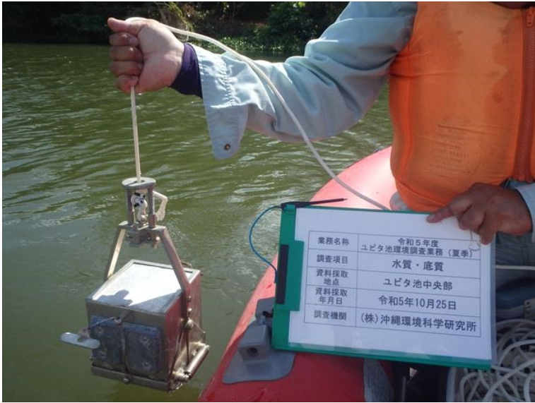
令和5年10月25日 夏季 水質・底質調査 試料採取状況（底質） エクマンバージ採泥器
