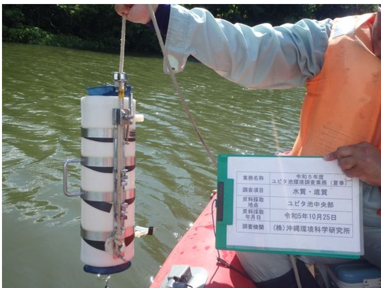
令和5年10月25日 夏季 水質・底質調査 試料採取状況（水質） バンドーン採水器
