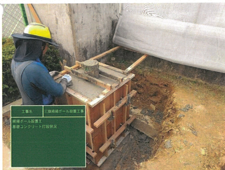
三旗掲揚ポール設置工 基礎コンクリート打設状況
