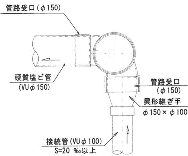
平面図 (上流がφ100mm)
