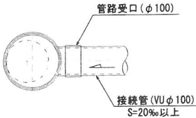
平面図
